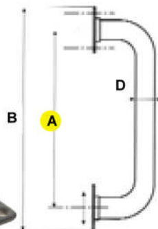
Art. 490 Tipo diritto Type droit Right model Tipo recto
