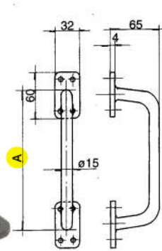
Art. 482 Tipo diritto Type droit Right model Tipo recto
