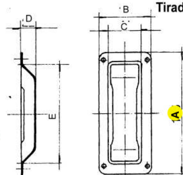
Art. 485/P Tipo piccolo Type petit Small size Tipo pequeno
