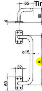
Art. 483 Tipo piegato Type plié bended model Tipo curvos
