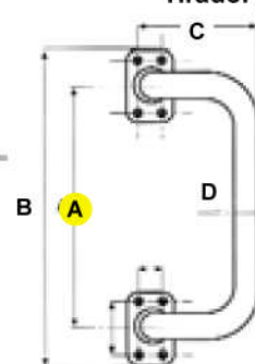
Art. 491 Tipo piegato Type plié bended model Tipo curvos
