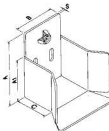
Art. 2120/M Art. 2120/P Incontro Butée Staple Encuentro
